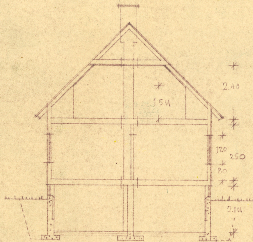
SNITT.
